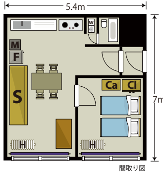
間取り図
